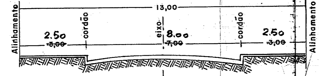
Perfil Transversal da RUA TIPO "B" Escala 1:100
