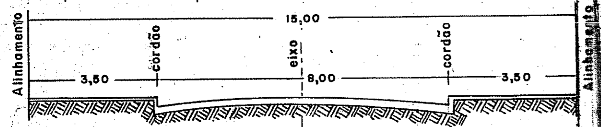
Perfil Transversal da RUA TIPO "A" Escala 1:100
