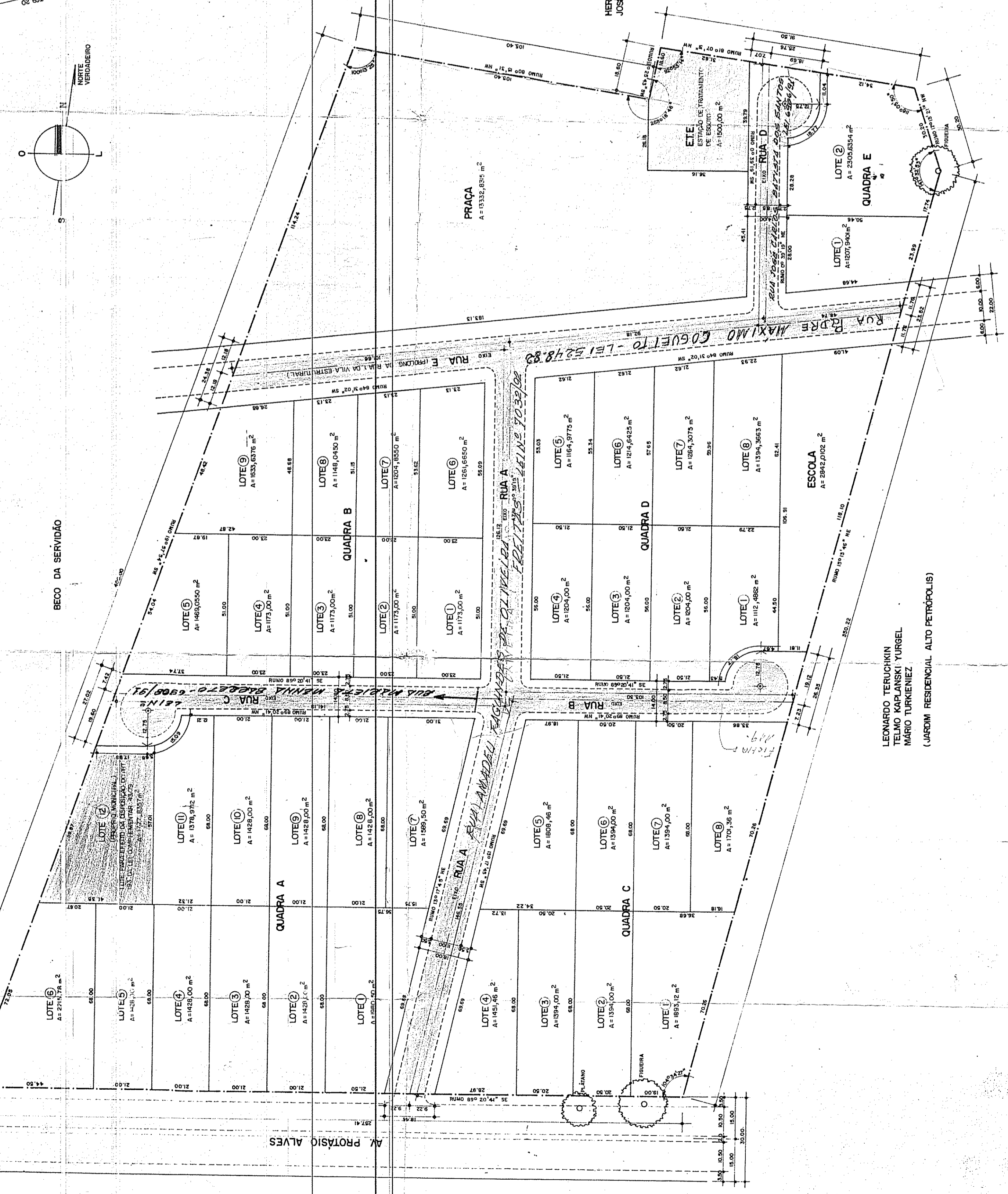
GABARITO DE RUAS ESCALA 1:500
