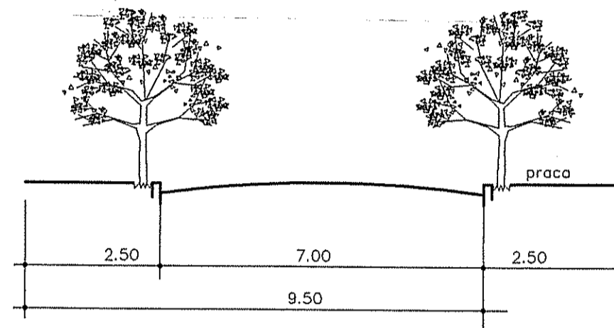
RUA DIRETRIZ 4061 PERFIL CONFORME ART 5o. DA LC. 547/06
