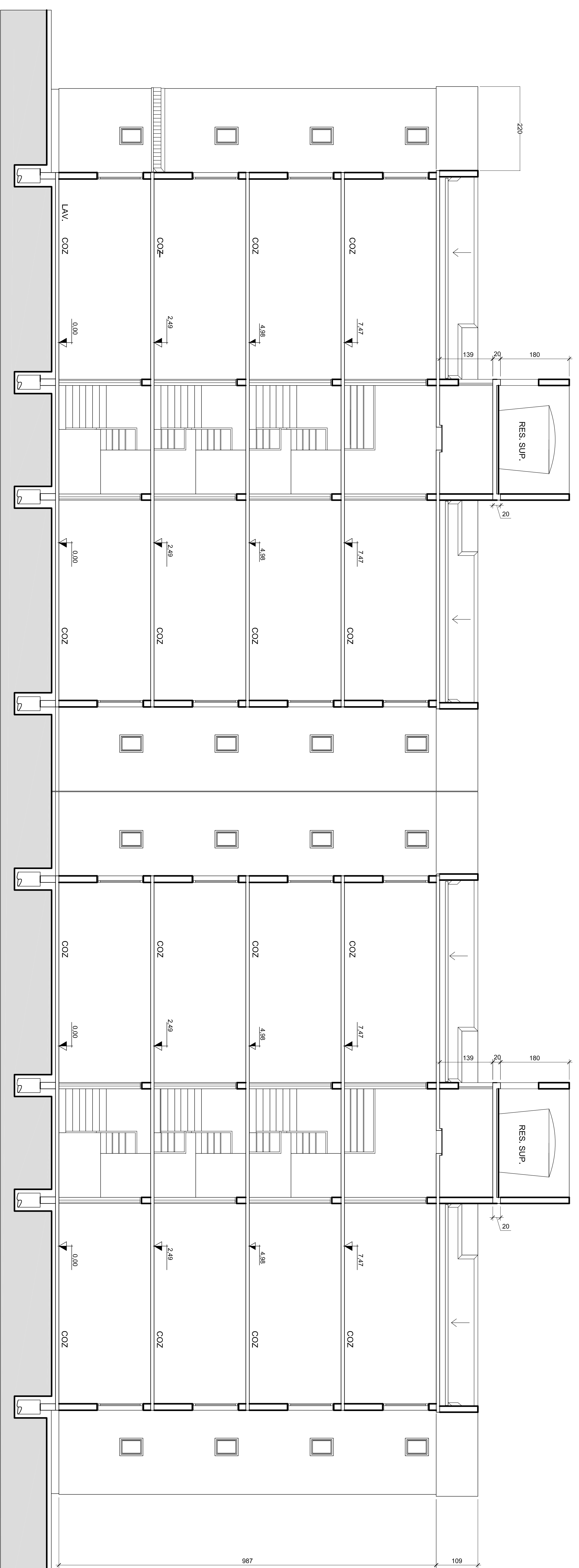
CORTE AA_ esc 1:50
