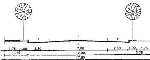
RV.II.3 VIA DE DISTRIBUI- ÇÃO DOMICILIAR, INTERIOR DE UTPs
