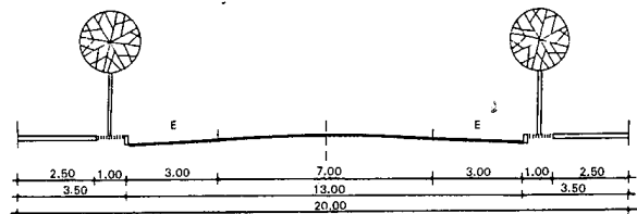
RV.II.2.1 VIA DE LIGA- ÇÃO E CONTORNO DE UTPs
