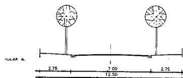
RV.III.4.2 VIA LOCAL DE ACESSO DOMICILIAR ALTERNATIVA PARA UTSE
