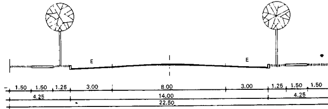
RV.II.1.1 VIA INDUSTRIAL DE DISTRIBUIÇÃO - PERFIL BÁSICO
