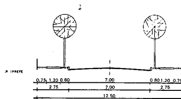
RV.III.4.1 VIA LOCAL DE ACESSO DOMICILIAR (PREFERENCIAL PARA HABITAÇÃO UNIFAMILIAR)
