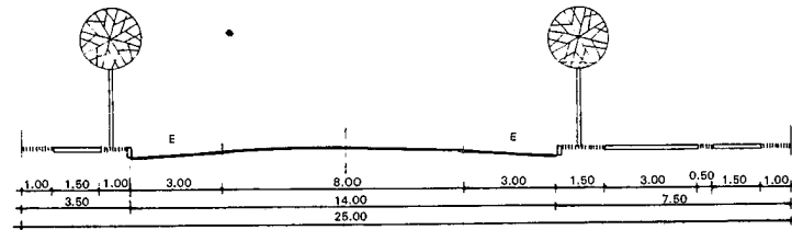
RV.II.1.2 VIA INDÚSTRIA DE DISTRIBUIÇÃO - PERFIL COM CICLOVIA
