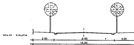
RV.III.3 VIA LOCAL DE ACESSO DOMICILIAR -EVOLUTIVA PARA RV.III.2
